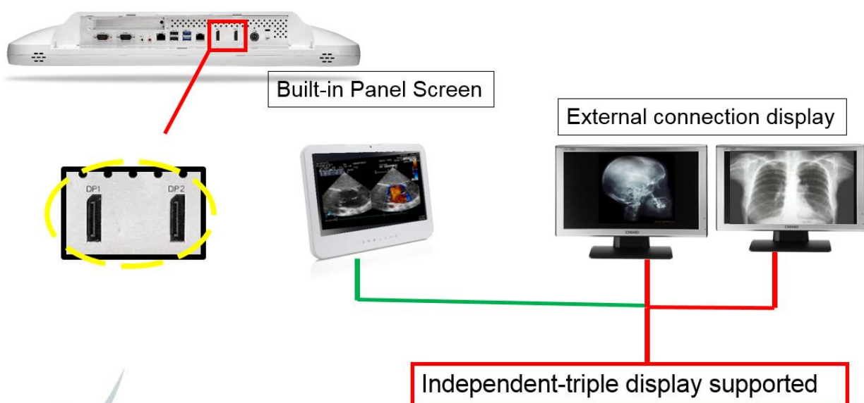
図： ディスプレイポート出力 x 2 ポートを利用することで独立した3つの画像を表示可能
