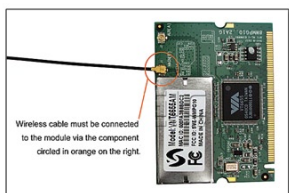
Mini-PCI
