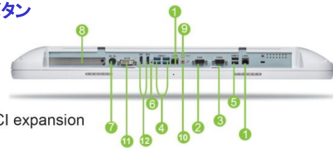
WMP-248/249のI/Oポート
